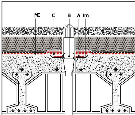
Det. DESAGÜE
