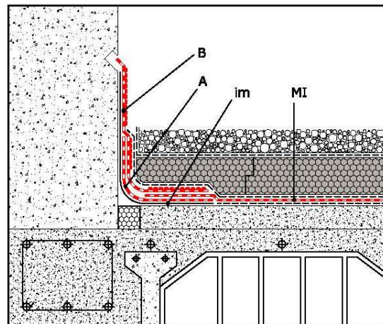
Det. ROZA
