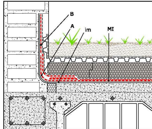
Det. RETRANQUEO
