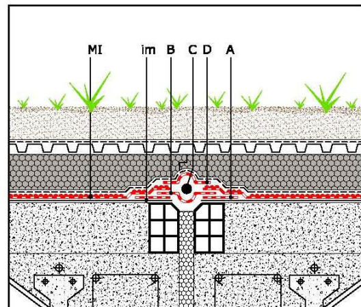
Det. JUNTA ESTRUCTURAL
