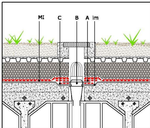
Det. DESAGÜE
