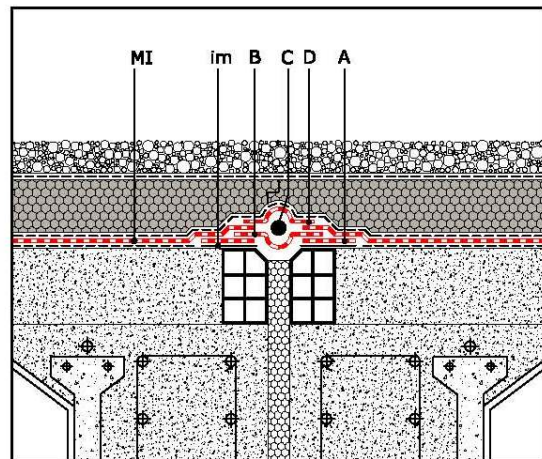
Det. JUNTA ESTRUCTURAL
